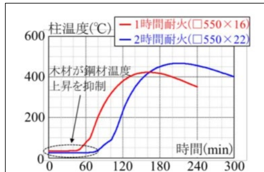
図 8.17 鋼材表面温度履歴
