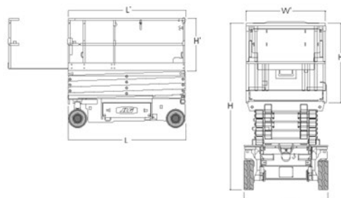
垂直式高所作業車
