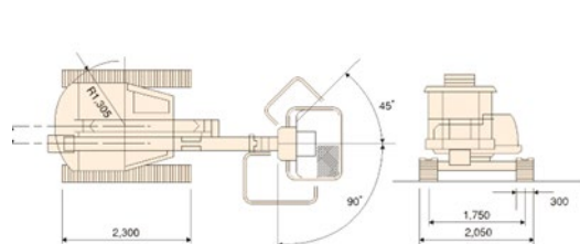
ブーム式高所作業車
